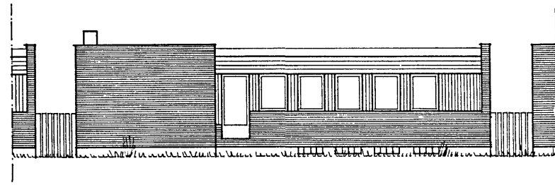
TRÄDGÅRDSFASAD
