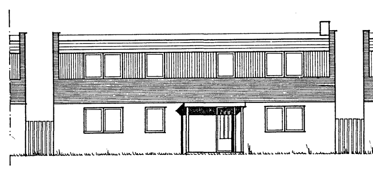
ENTRÉFASAD
